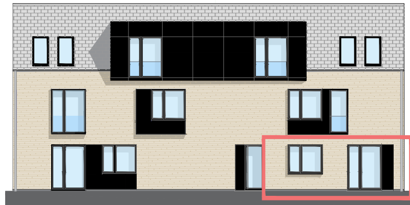
VOORGEVEL
