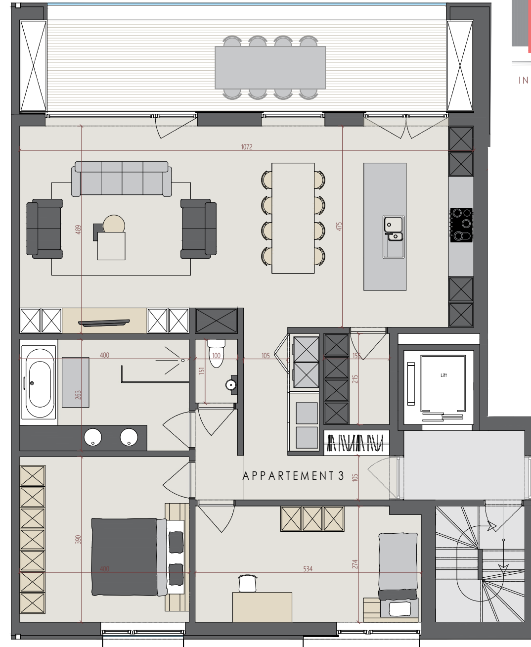
EERSTE VERDIEPING
