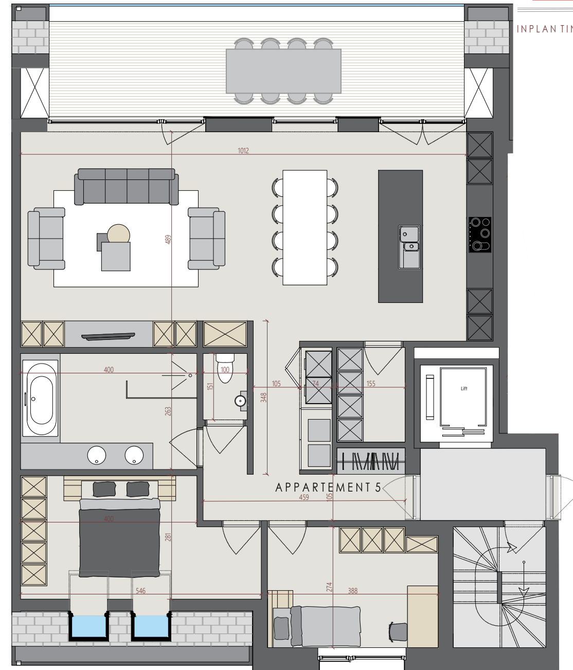
TWEDE VERDIEPING
