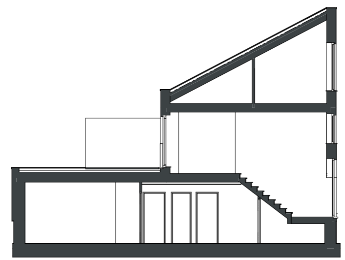
PRINCIPEDOORSNEDE
