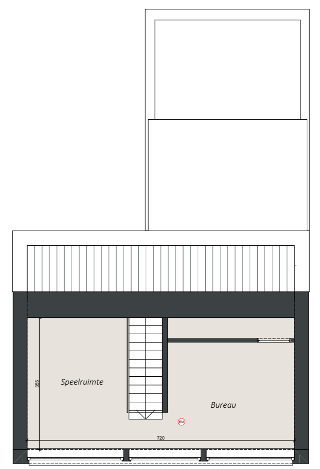
TWEDE VERDIEPING
