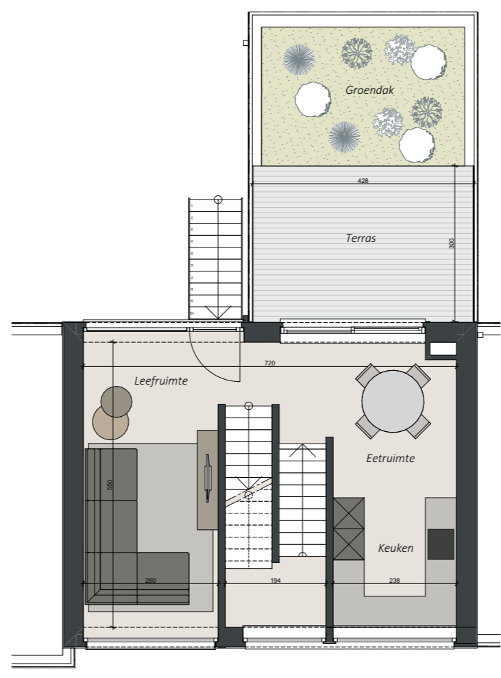
EERSTE VERDIEPING
