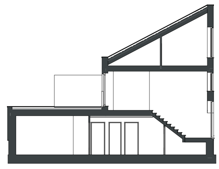
PRINCIPEDOORSNEDE
