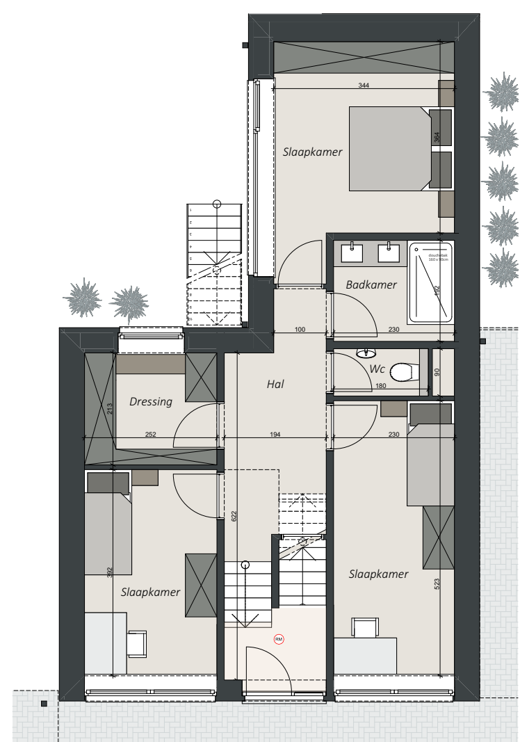
GELIJKVLOERS
